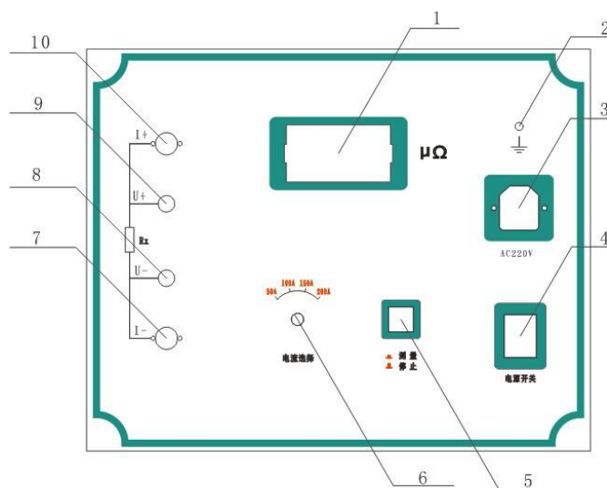
图一 面板布局图
